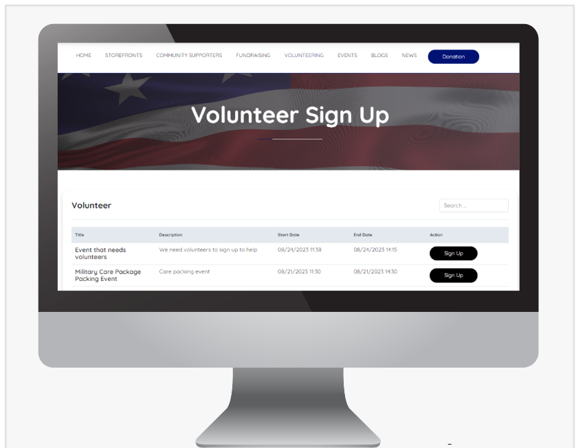
501Techstack Screenshot
